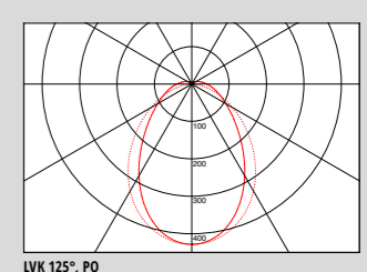
LVK 125°, PO
