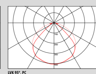
LVK 95°, PC
