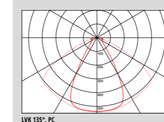
LVK 135°, PC
