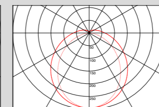
LVK 80°, PO
